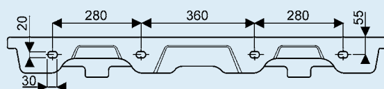
Fixation plan de 96
