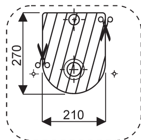
Bonde à écoulement libre
