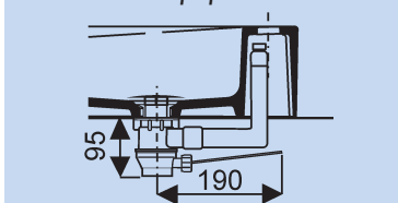
Bonde à trop-plein invisible
