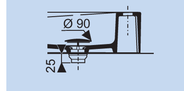
Bonde à écoulement libre
