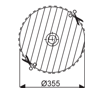
Vasque Uzès 001647 00 xxx (découpe du plan : Ø 355 mm)
