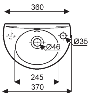
Lave-mains 001702 00 xxx
