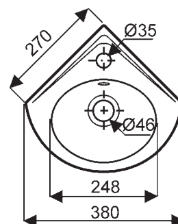
Lave-mains 001712 00 xxx
