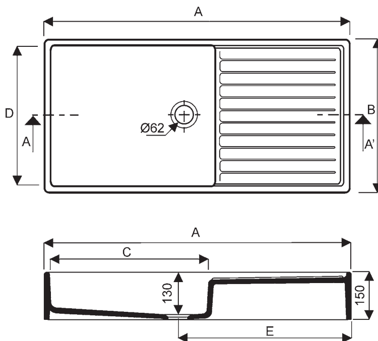
Coupe AA'
