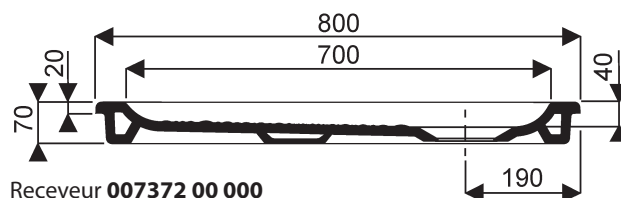
Receveur 007372 00 000
