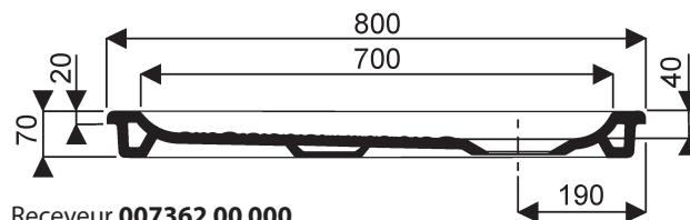
Receveur 007362 00 000
