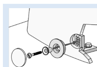
Détail des fixations cachées fournies
