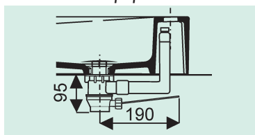
Bonde à trop-plein invisible
